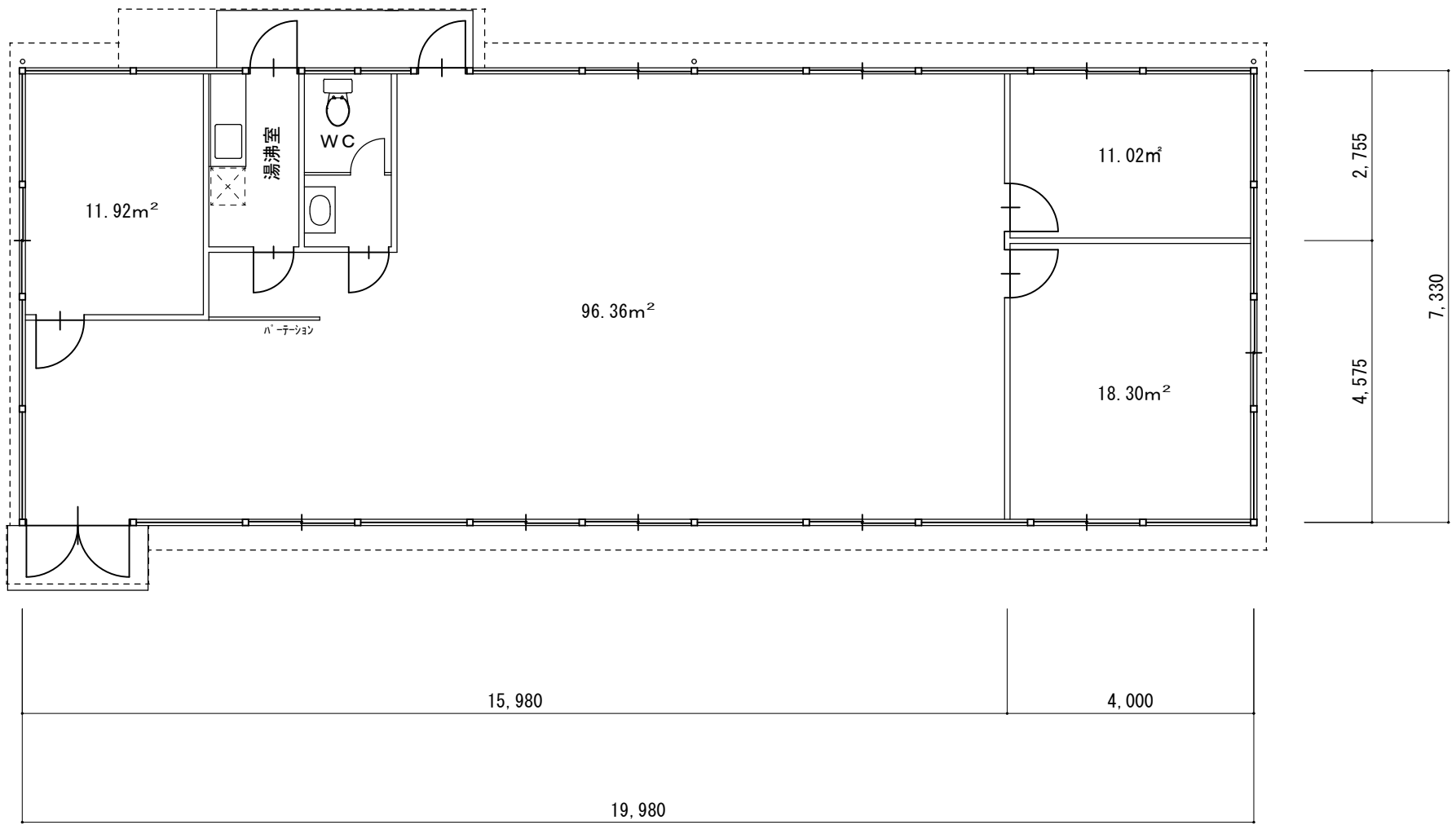
1 階平面図 1/100
